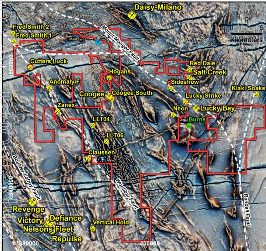
Aeromagnetics Grey Scale TMI3VD
