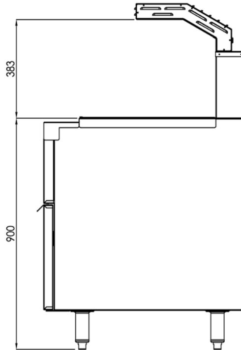
End Elevation
